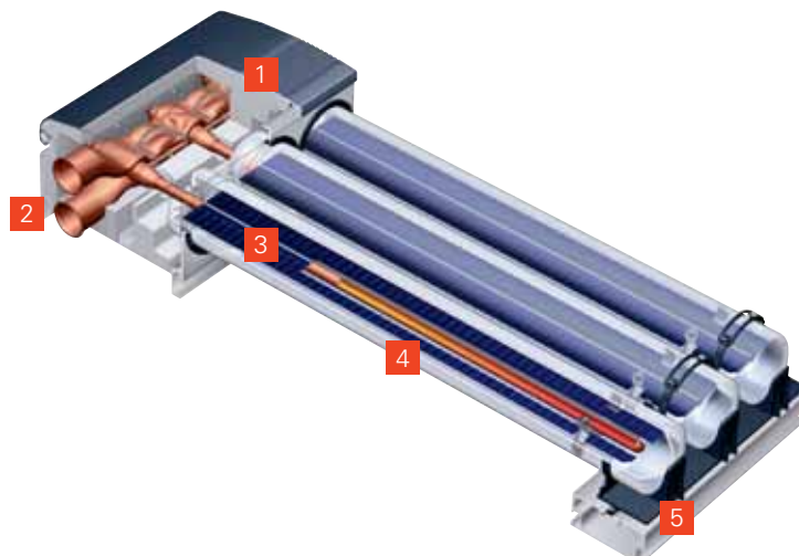
Einfache Installation und schnelle Absorberausrichtung durch Winkelanzeige an den Röhrenaufnahmen
